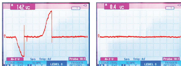
Abb. 2: Ableitung der Spannung aus der Motorwelle vor (links) und nach (rechts) der Montage des AEGIS® SGR Lagerschutzrings.
